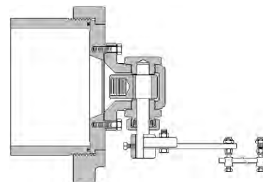
8" поворотно-тяговый блок с быстроразъемным соединением HUTA
